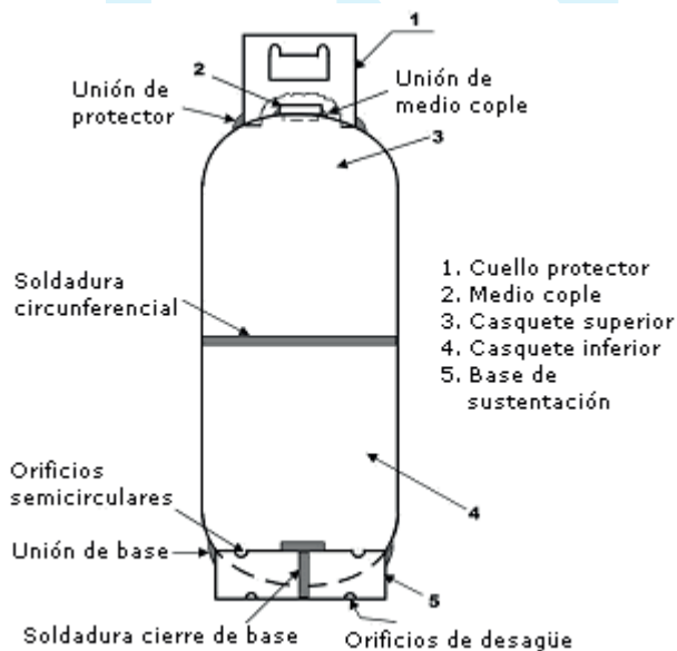
Recipiente Clase I, Tipo Semicapsulado
