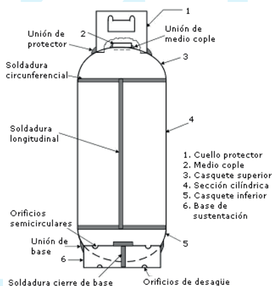
Recipiente Clase I Tipo Común
